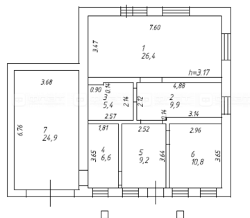
ПОЭТАЖНЫЙ ПЛАН ОБЪЕКТА План 1 этажа
