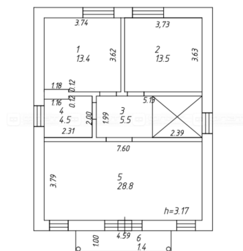
ПОЭТАЖНЫЙ ПЛАН ОБЪЕКТА План 2 этажа
