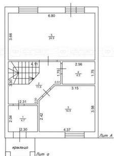
План 1 этажа
