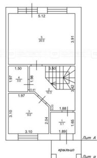
План 1 этажа
